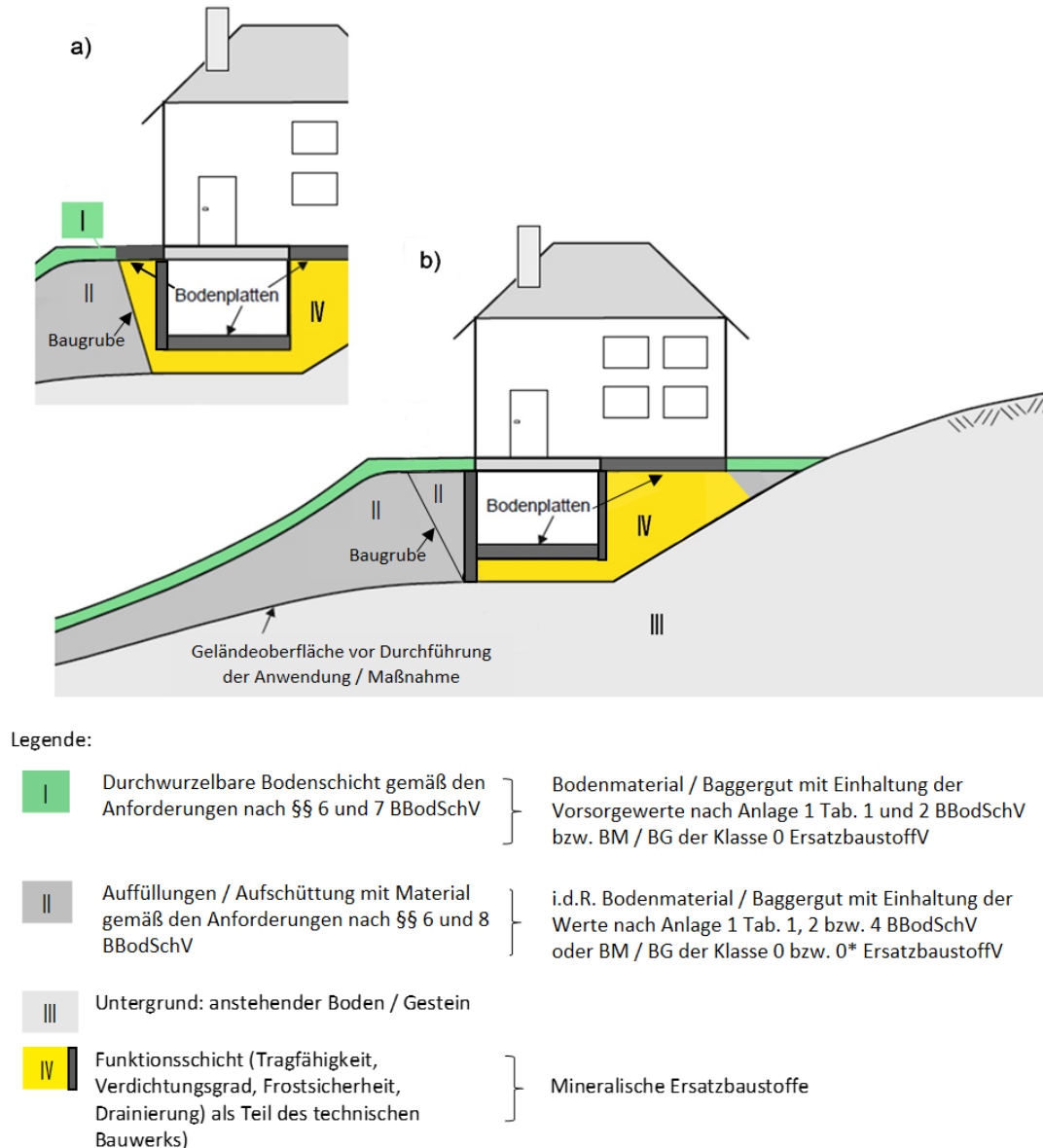
Abbildung 6: Prinzipskizze - Bodenähnliche Anwendung als Geländeauffüllung und Unterbau von Gebäuden mit Verfüllung von Baugruben (a) mit und (b) ohne gebundene oder ungebundene Deckschicht (verändert nach LfU RP (2020)).
